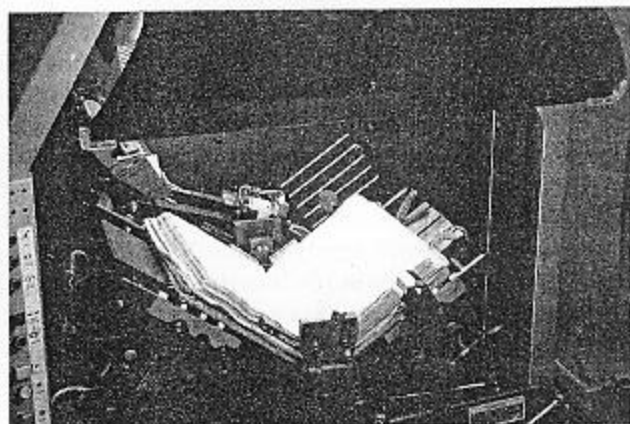
Процесс сканирования
